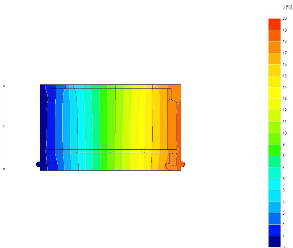
Izotermie, strumień cieplny, temperatury. Przekrój Profila: VG i V , 1 - 30mm.
